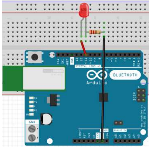
Figura 14: Circuito com um resistor (220Ω) e um LED Fonte: Do autor.
