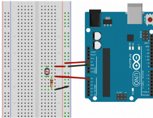
Figura 17: Divisor de tensão com LDR e resistor de 10kΩ
