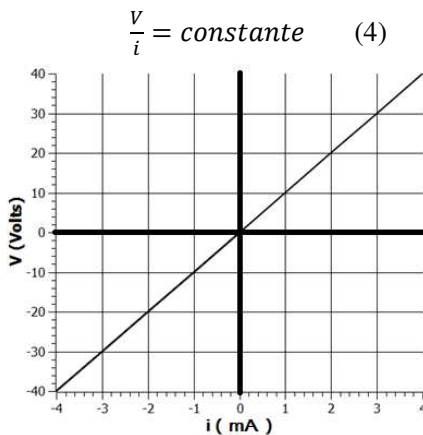
Figura 2: Gráfico V \times i de um resistor ôhmico de 10k\Omega .
