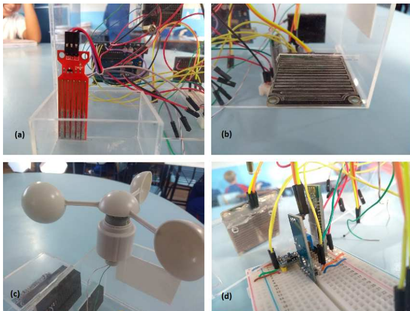
Figura 26: Pluviômetro (a) sensor de chuva (b) anemômetro (c) módulo Bluetooth (d) montado pelo grupo 2
