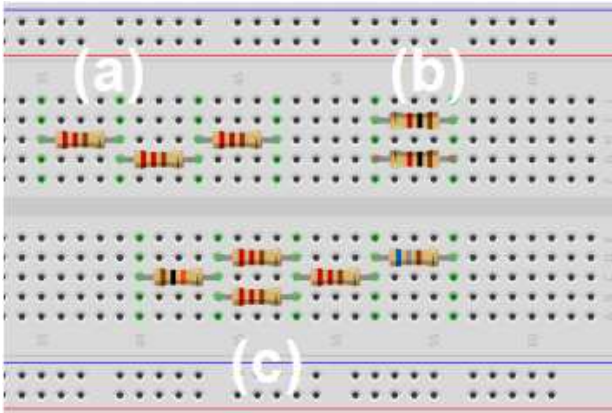
Figura 10: Exemplos de associação em série (a), paralelo (b) e mista (c) Fonte: Do autor
