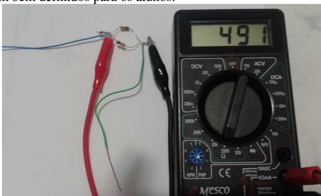
Figura 13: Medindo resistência elétrica
