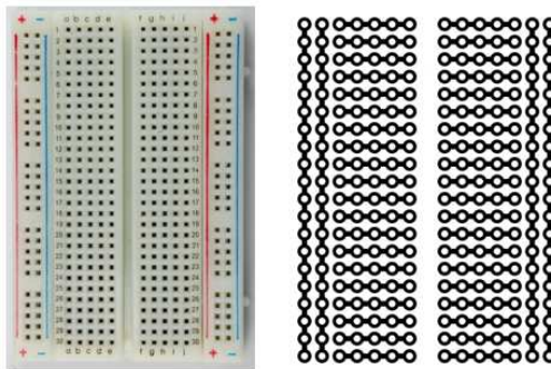
Figura 10: Esquema de ligação de uma protoboard
