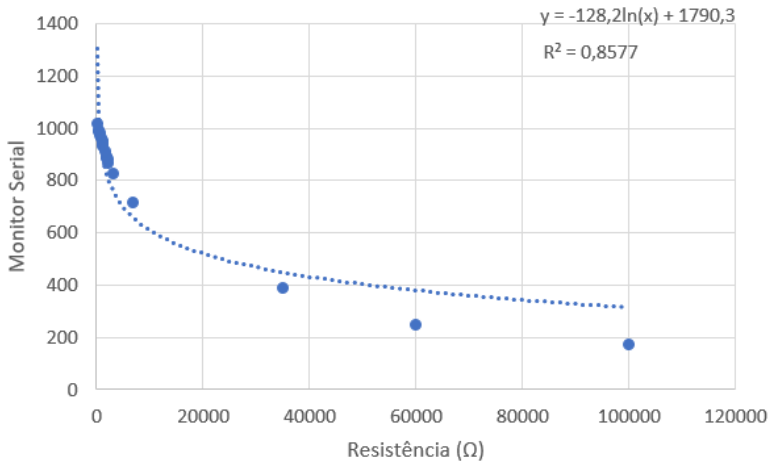
Figura 22: Monitor serial x Resistência (Ω) Fonte: Do autor
