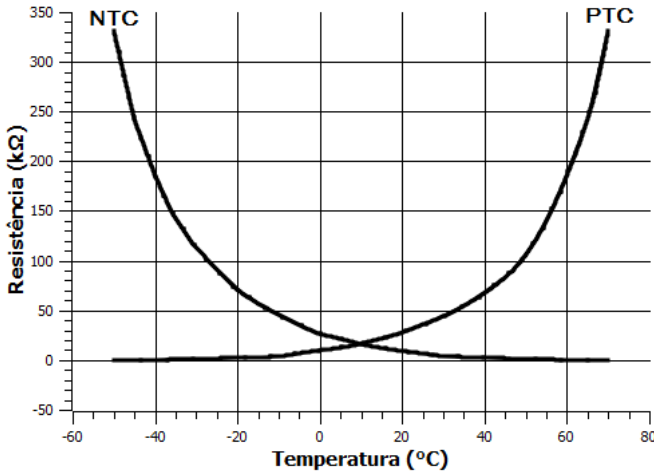
Figura 6: Gráfico Resistência x Temperatura nos termistores NTC e PTC
