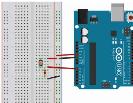
Figura 19: Sistema divisor de tensão com um LDR e um resistor de 10k\Omega
