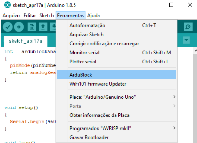
Figura 17: Configurando o Ardublock na IDE do Arduino.
