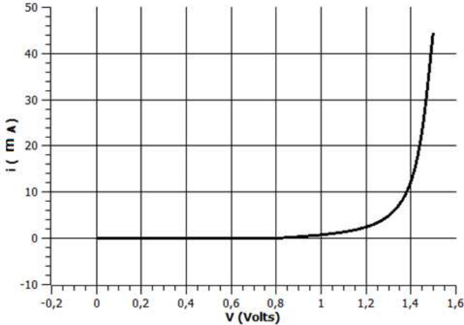
Figura 4: Gráfico i \times V de um resistor não-ohmico do tipo LED Fonte: Do autor
