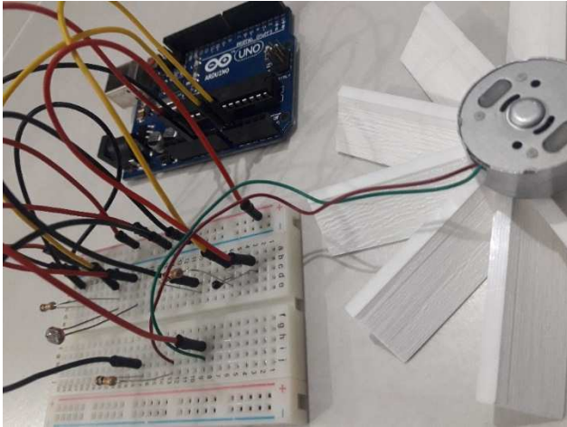
Figura 23: Sensor de luz, temperatura e velocidade Fonte: Do autor
