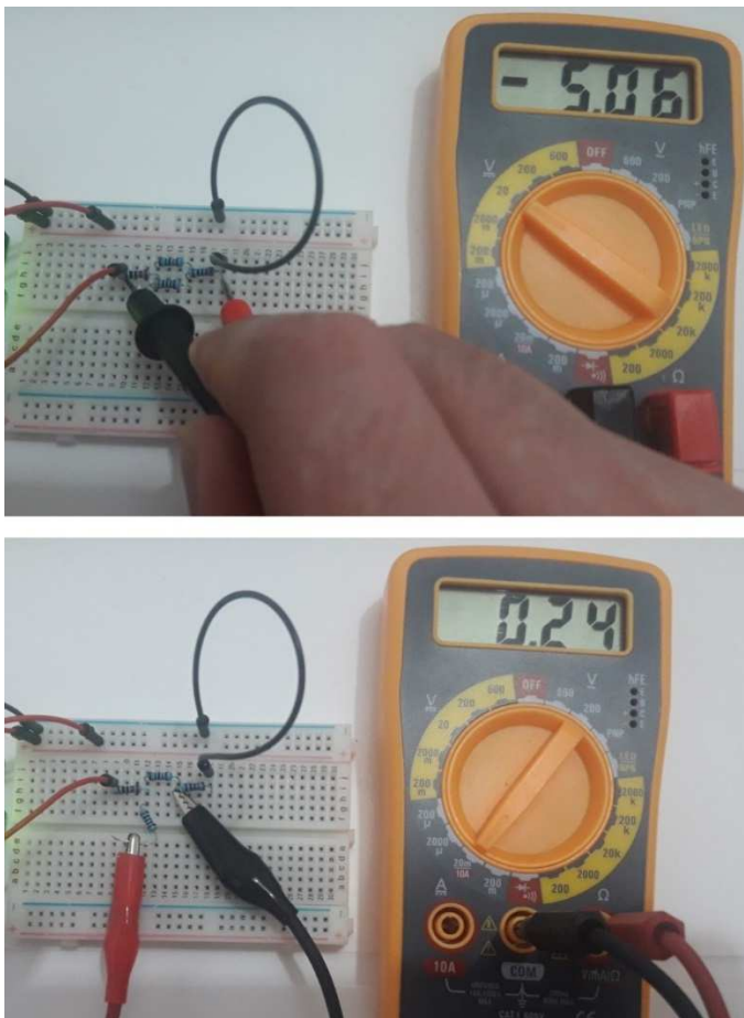
Figura 12: Multímetro associado em paralelo e em série no circuito, respectivamente Fonte: Do autor.
