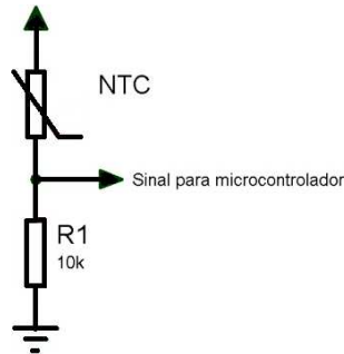
Figura 7: Divisor de tensão
