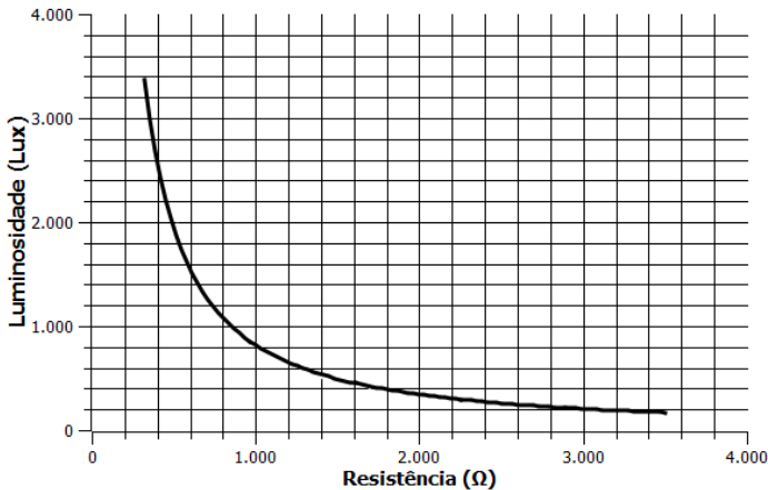
Figura 9: Gráfico Luminosidade x Resistência Fonte: Do autor
