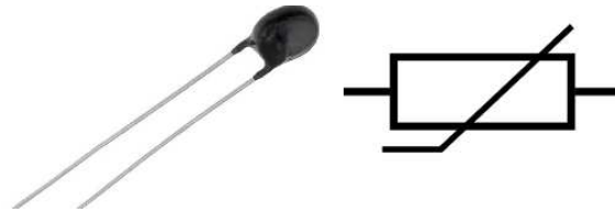
Figura 5: Termistor e sua representação em esquemas eletrônicos Fonte: http://www.retroamplis.com/Termistor-ceramico-5mm-NTC . Visualizado em ago. 2017. Visualizado em ago. 2017
