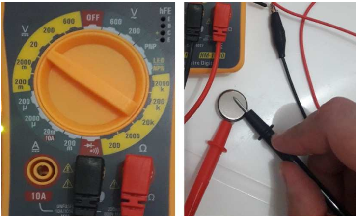
Figura 1: Medindo a tensão de uma bateria de 3V em corrente contínua Fonte: Do autor
