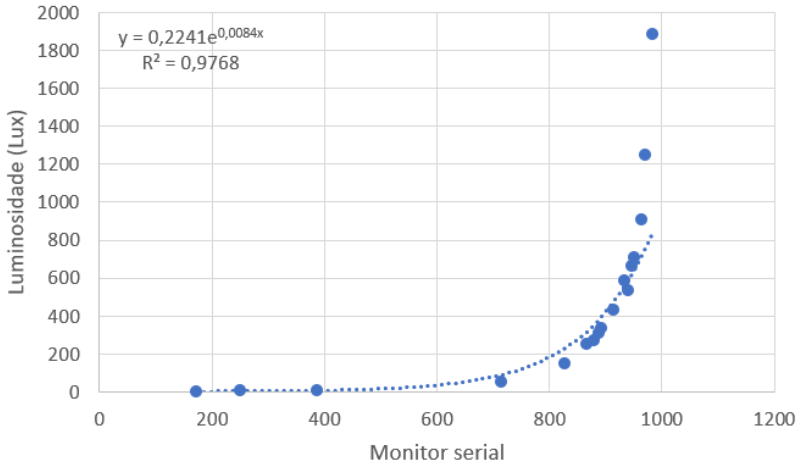
Figura 23: Luminosidade (Lux) x Monitor Serial (m) Fonte: Do autor
