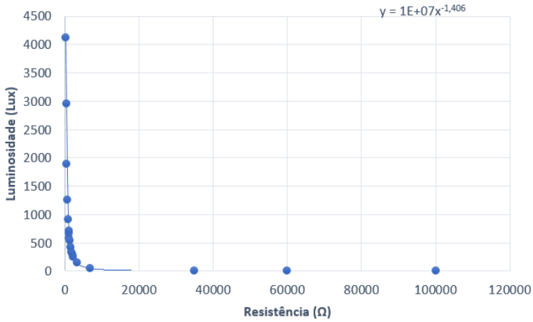
Figura 21: Gráfico Luminosidade (Lux) x Resistência (Ω) Fonte: Do autor
