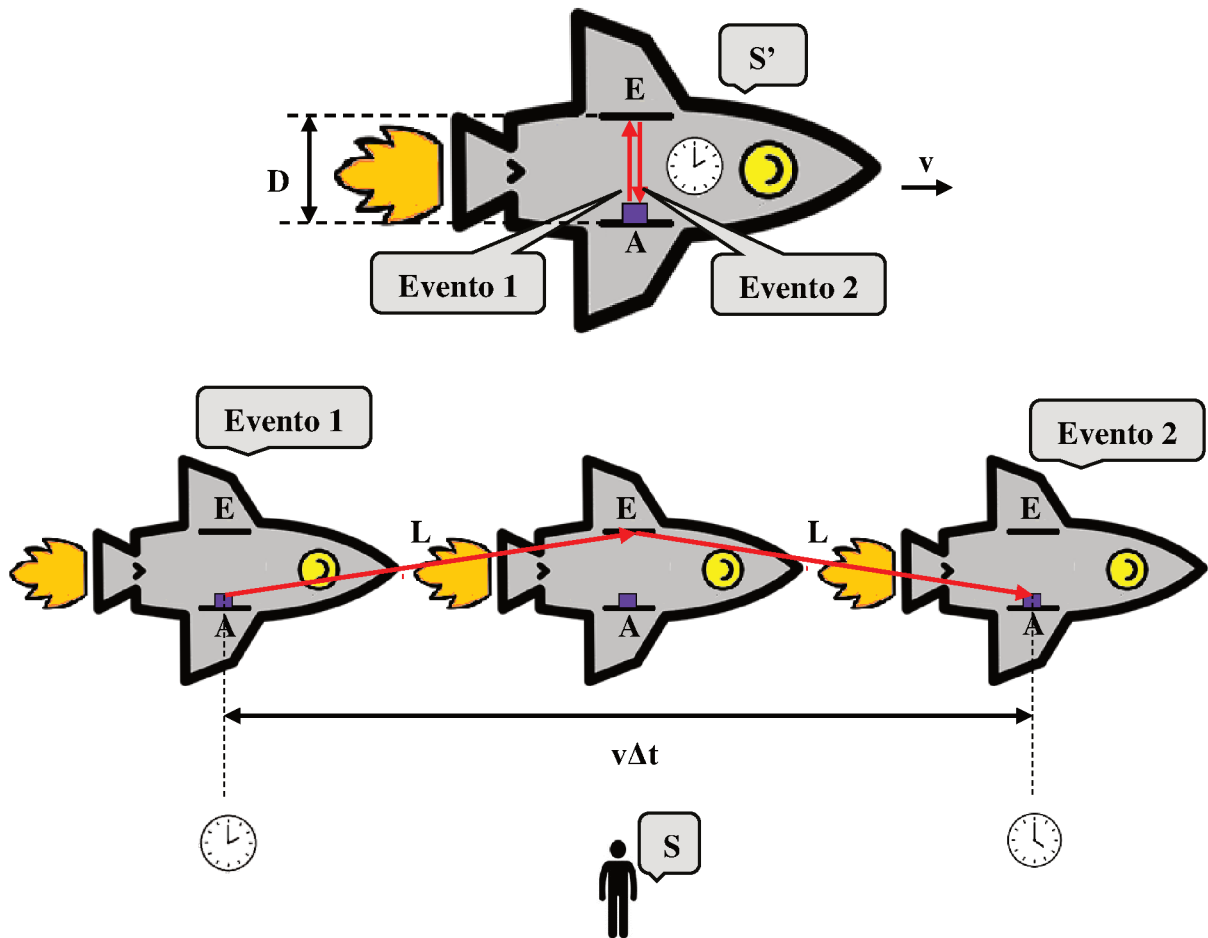
Figura 9 - Análise da Dilatação Temporal
