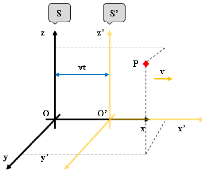
Figura 3 - Translação (na direção +x) de um sistema inercial S' em relação a um sistema inercial em repouso, S.
