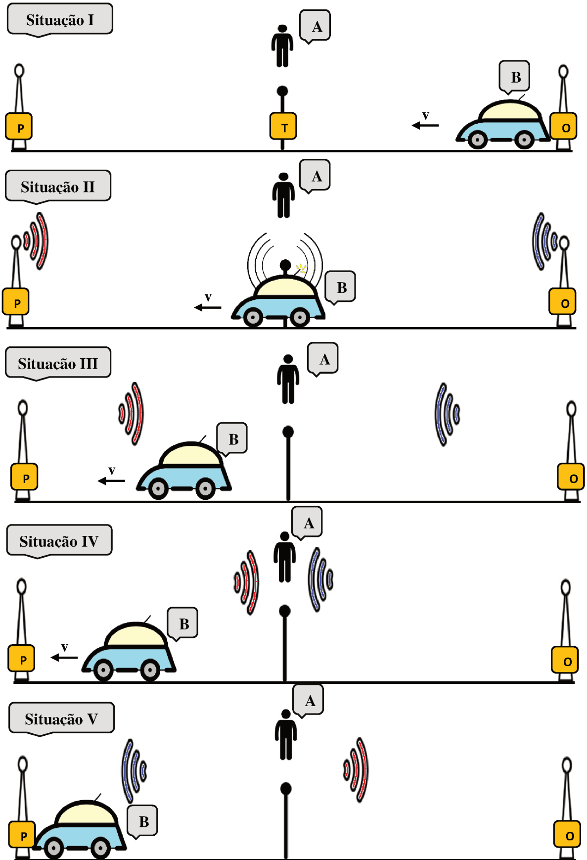
Figura 8 - Análise da Simultaneidade
