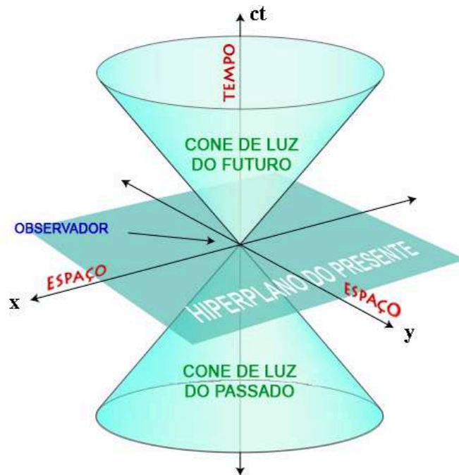
Figura 5 - Representação da estrutura do espaço-tempo no espaço de Minkowski.
