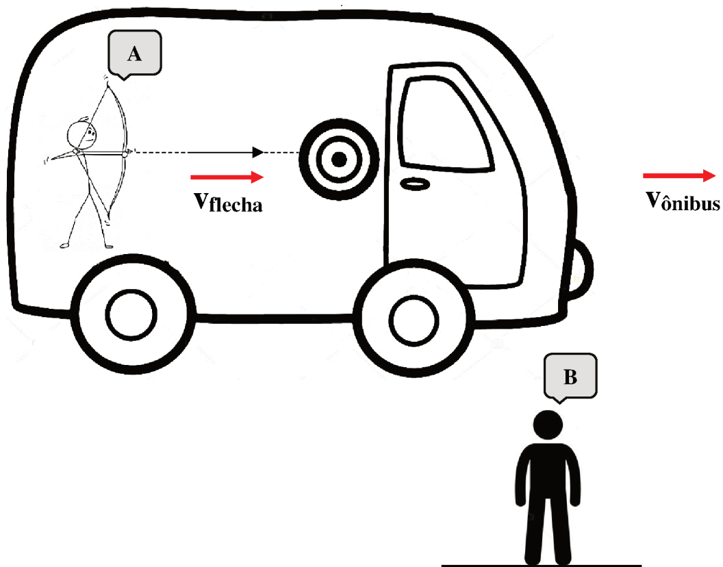
Figura 4 - Movimento relativo e composição (adição) de velocidades em dois referenciais inerciais
