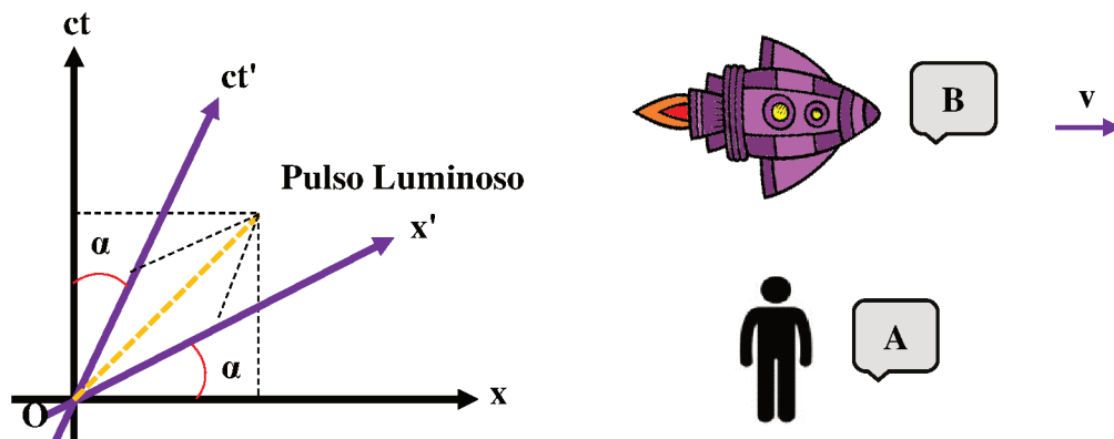
Figura 7 - Análise do Espaço de Minkowski
