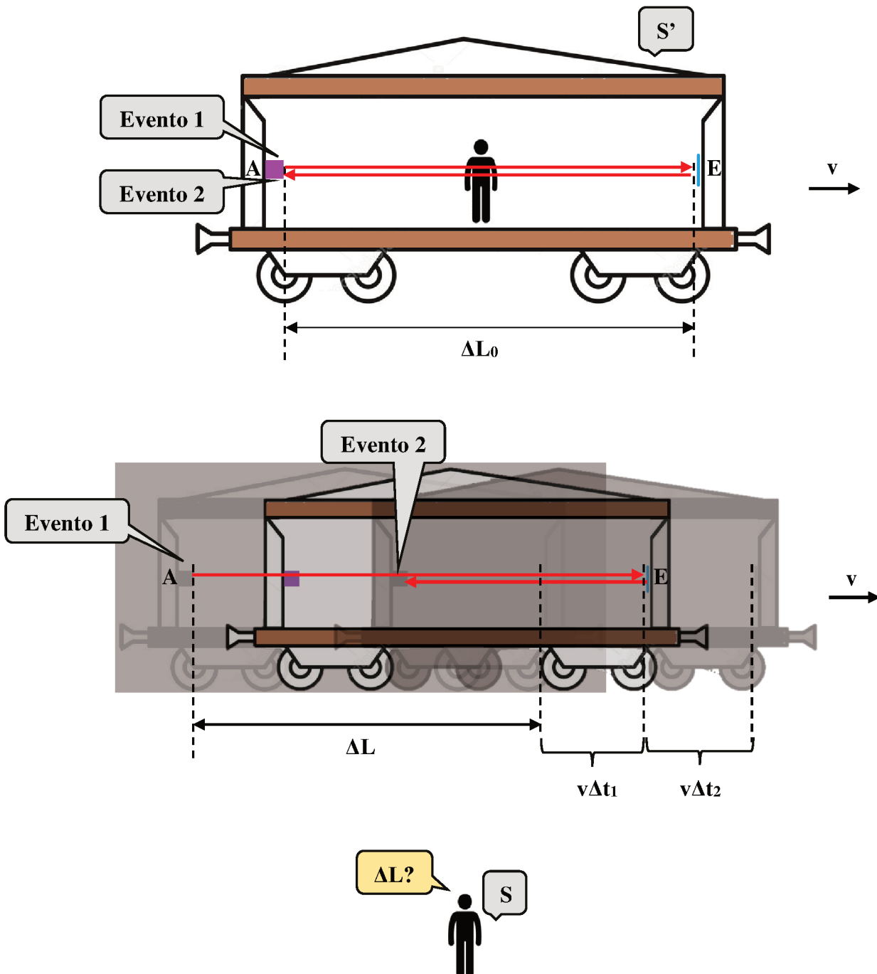
Figura 10 - Análise da Contração do Comprimento
