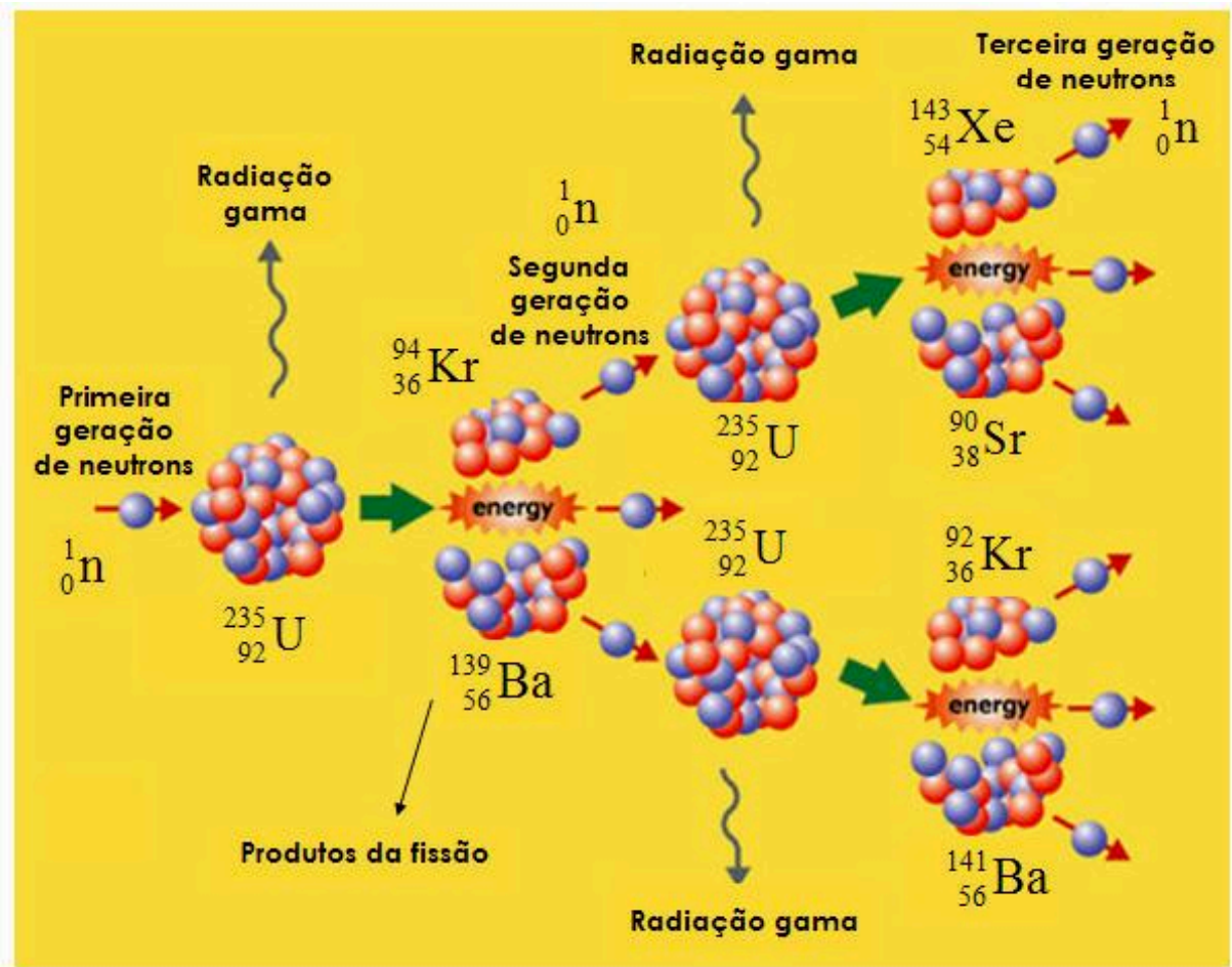
Figura 2 - Reação em Cadeia Urânio-235
